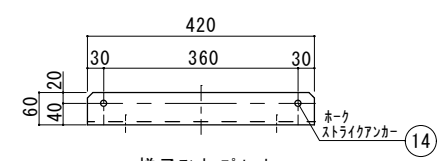
梯子アンカープレート D 矢視
