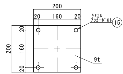
支柱プレート C 矢視
